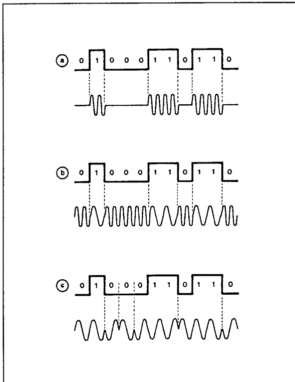
Fig. 61: Drie vormen van modulatie
