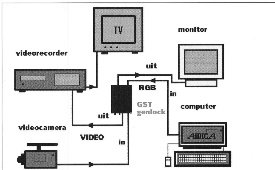
4. Aansluitschema
