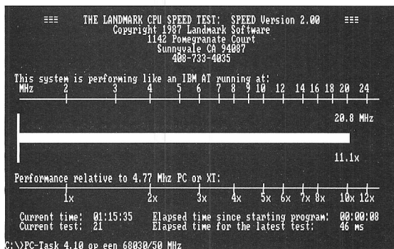
De Landmark-test houdt het bij PC-Task op een snelle AT.
