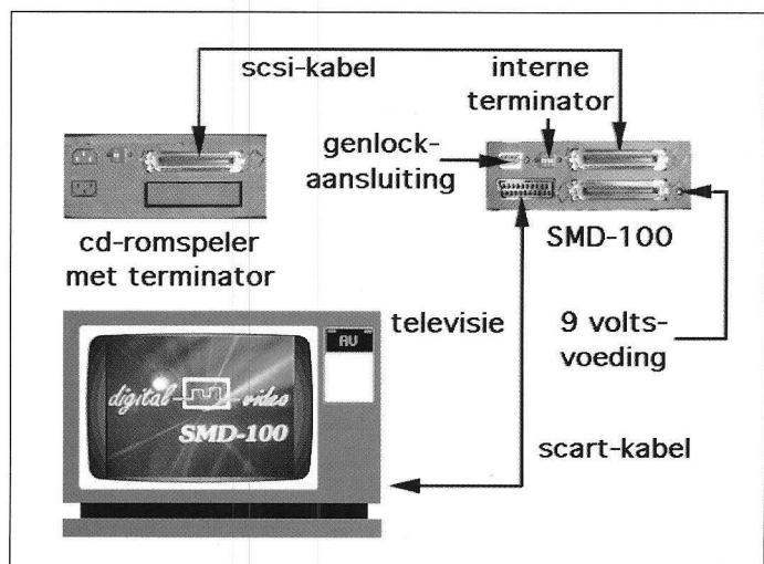
Figuur 2: Het aansluitschema van HiSoft's SMD-100.
