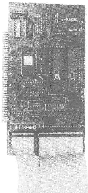
Kronoscontroller
